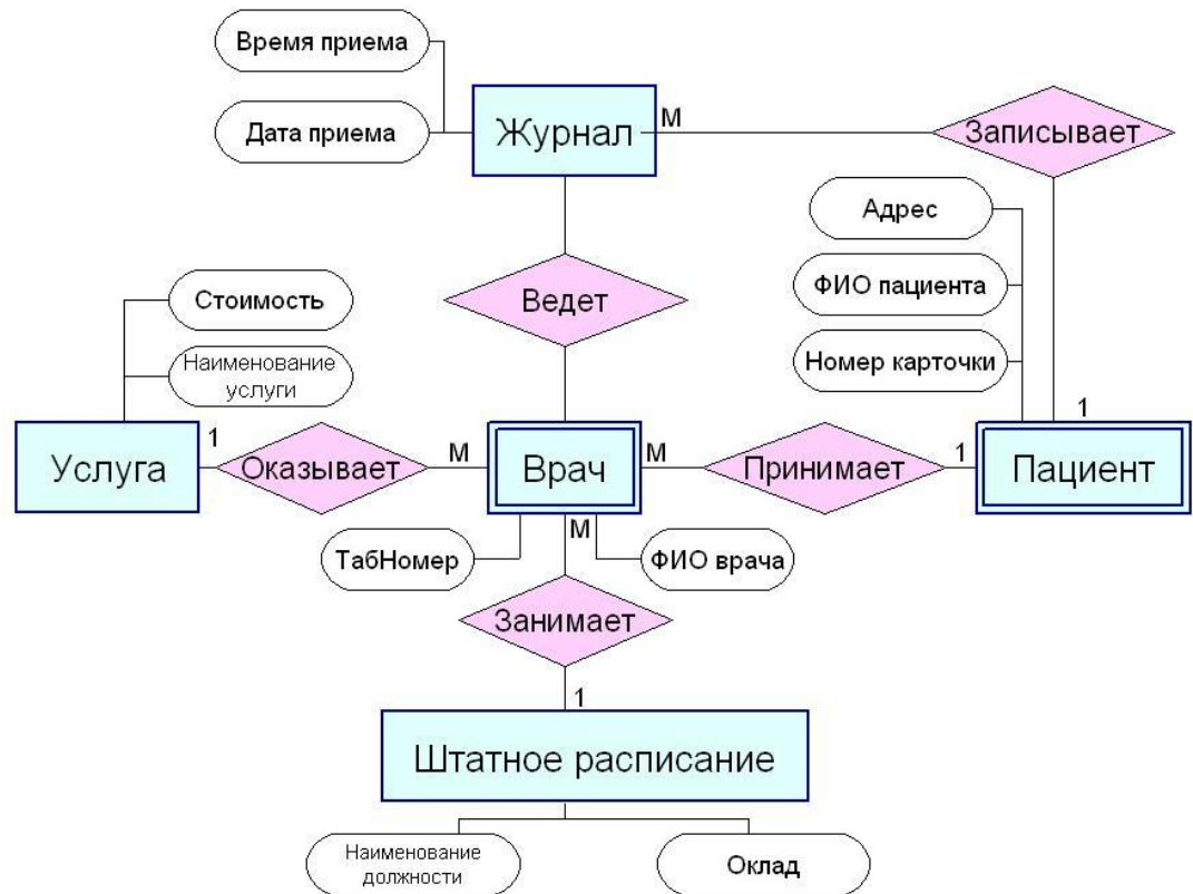
Рис.20. Пример ER-диаграммы
